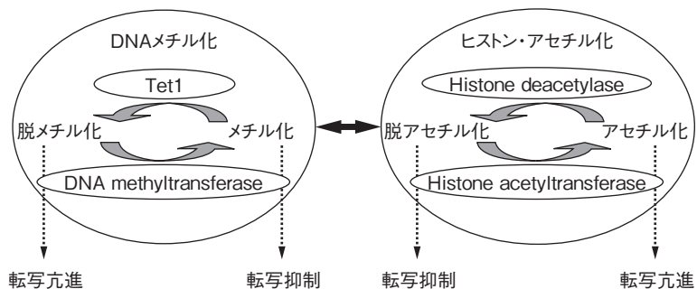
図3 エピジェネティクスによる遺伝子の転写調節機構
